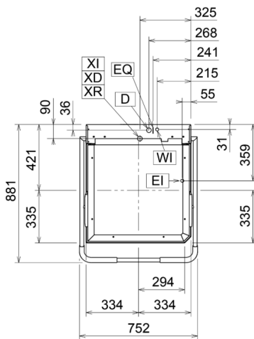
Päältä
